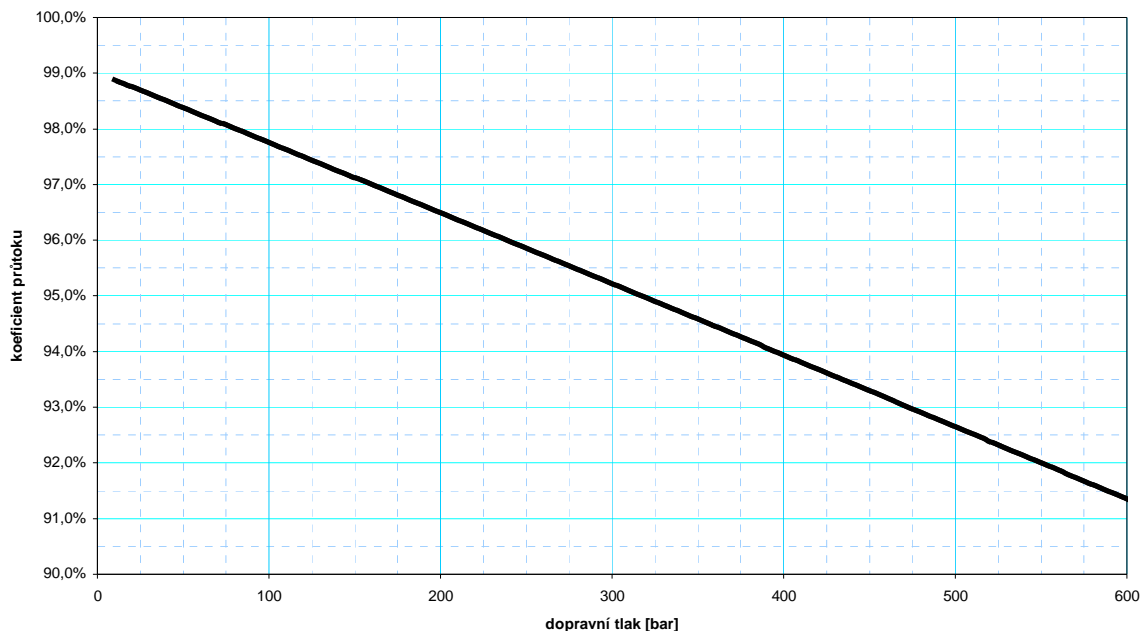
graf 1 : koeficient průtoku
