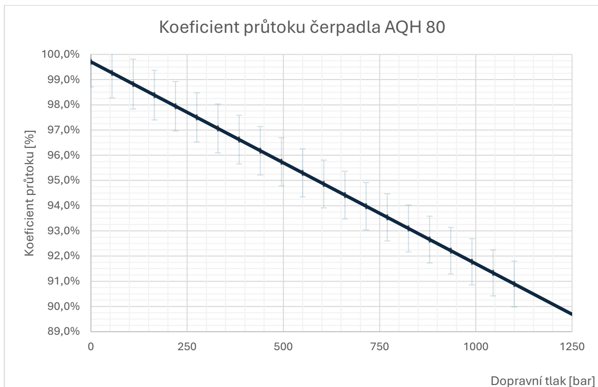
Obrázek 1: Koeficient průtoku čerpadla AQH 80
